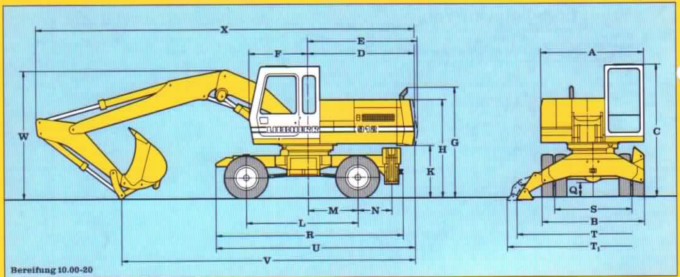
Bereifung 10.00-20
