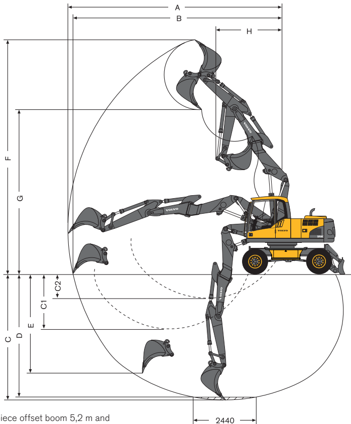
2-piece offset boom 5,2 m and dipper arm 2,0 m, 2,45 m, 2,6 m, 3,1 m
